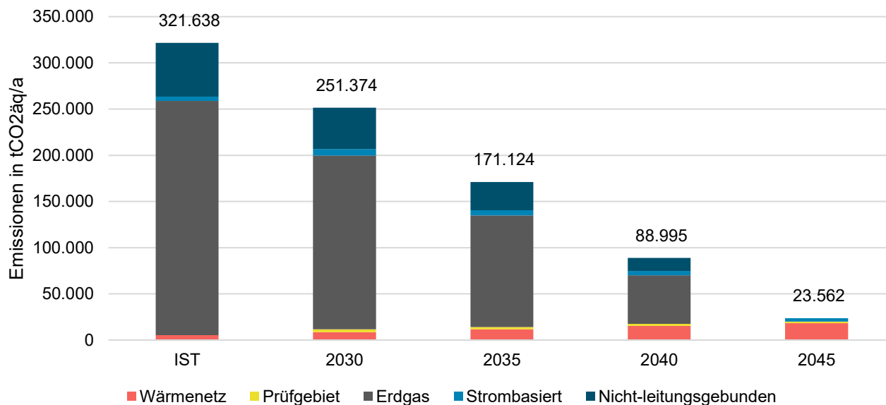
Abbildung 22: Treibhausgasemissionen der Energieträger in CO 2 äq/a bis 2045
