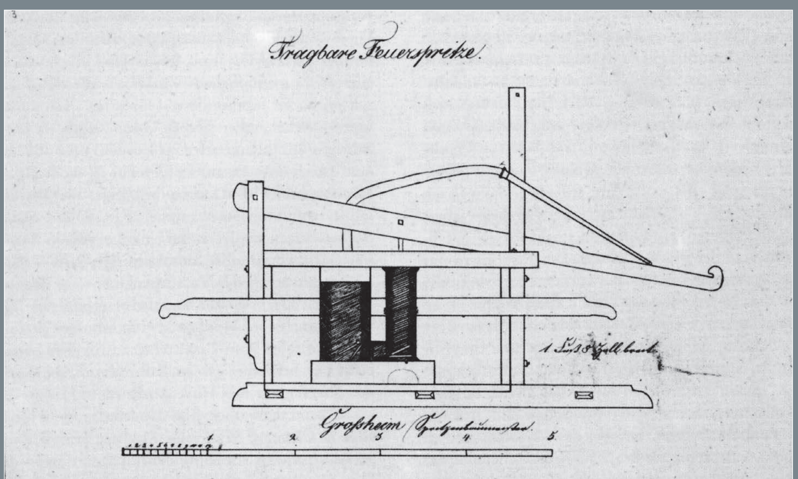
Feuerspritze aus Mitte des 18. Jahrhunderts | Stadtarchiv Hamm
